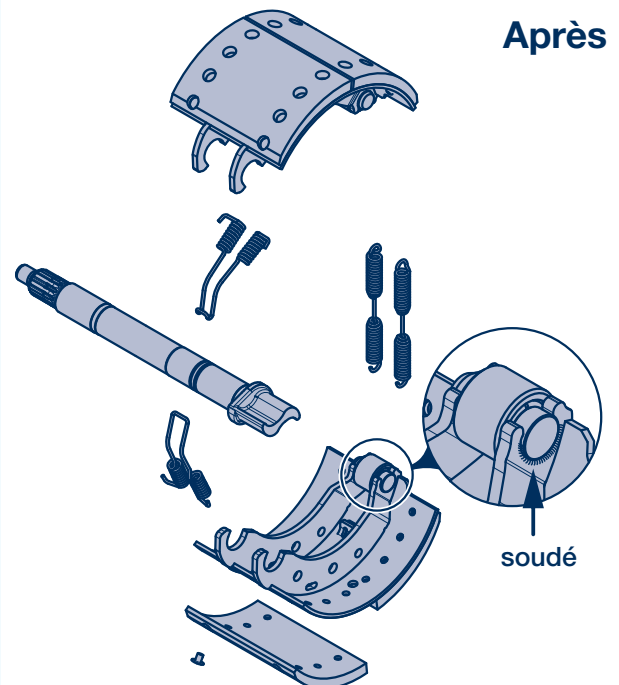
Mâchoire de frein : 05.005.79.34.1 Kit de réparation : 09.801.09.35.0
