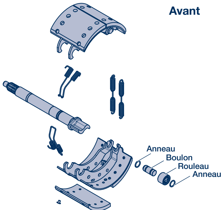
Mâchoire de frein : 05.091.14.77.1 (toujours valable pour les essieux 9 t avec SN 3020)
