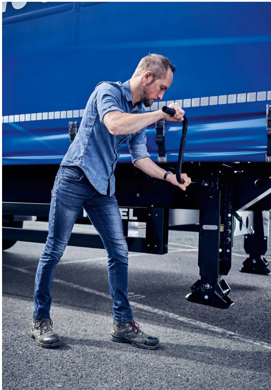
Die BPW Deichselstütze im Einsatz
