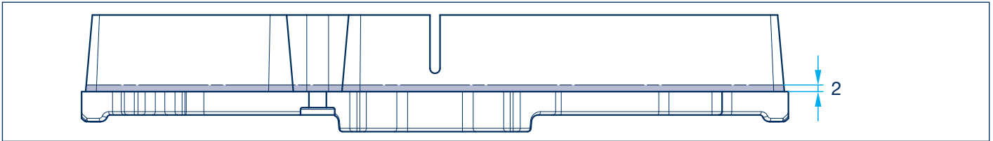
Bild 2: Kritischer Bereich der Belaganbindung, in diesem sind keine Ausbrüche oder Ablösungen zulässig.
